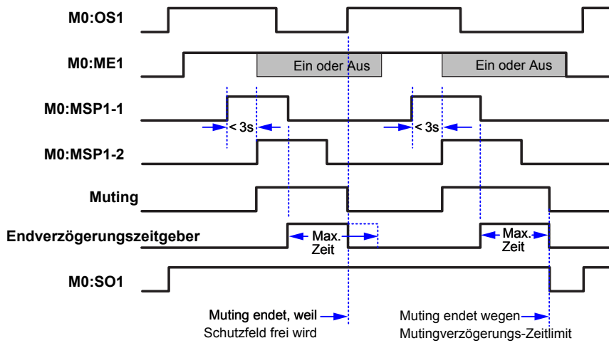
Abbildung 77. Zeitablauf-Diagramm: Unidirektionaler Muting-Block, ein Muting-Sensorpaar
