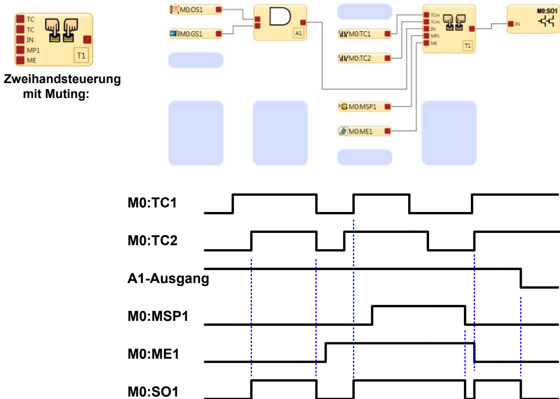
Abbildung 87. Muting-Optionen für Zweihandsteuerungen
