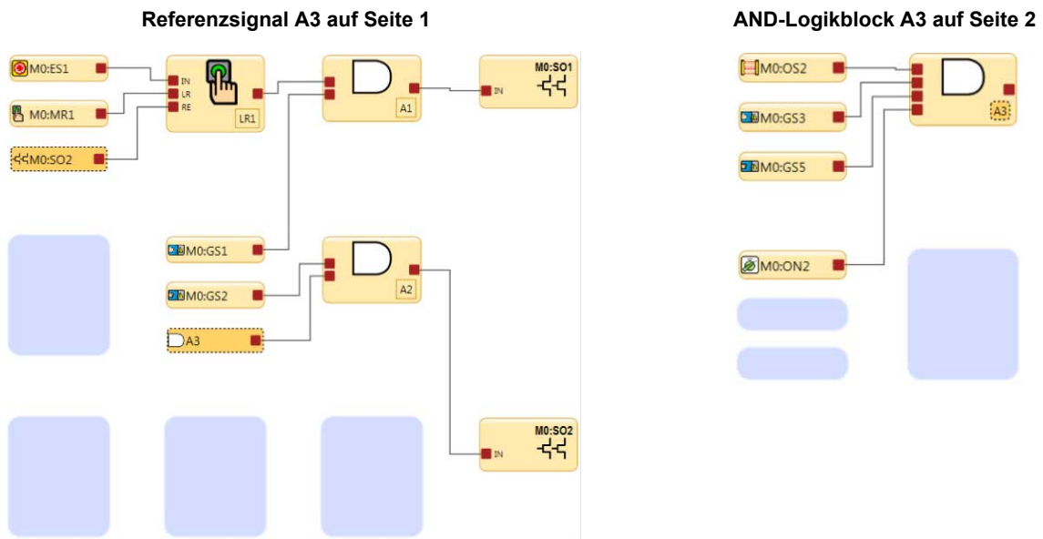
Abbildung 71. Latch-Reset und referenzierter Sicherheitsausgang und AND-Block
