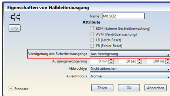
Abbildung 32. Auswahlbeispiel für Sicherheitsausgangsverzögerung: Ausschaltverzögerung
