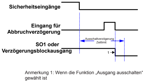
Abbildung 27. Sicherheitseingang verbleibt im Stopp-Modus
