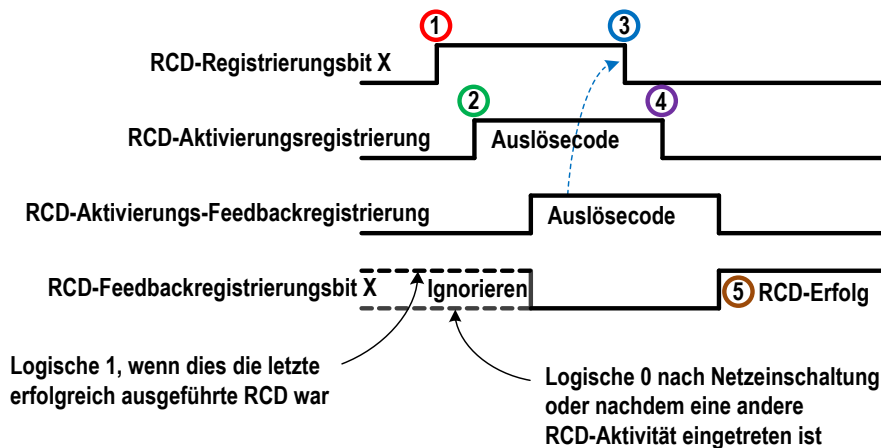
Abbildung 25. Virtuelle Reset- oder Abbruchverzögerungssequenz (RCD) - Feedbackmethode
