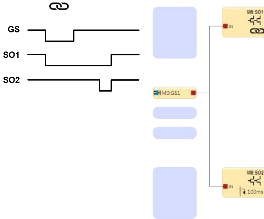
Abbildung 34. Zeitablauf-Diagramm: Verkettete Sicherheitsausgänge
