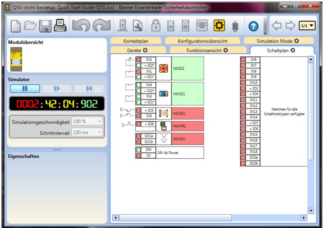
Abbildung 113. Simulationsmodus: Registerkarte Schaltplan
