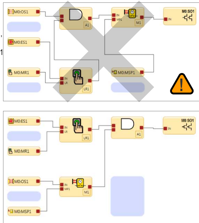
Abbildung 81. Not-Aus-Schalter und Muting-Funktion
