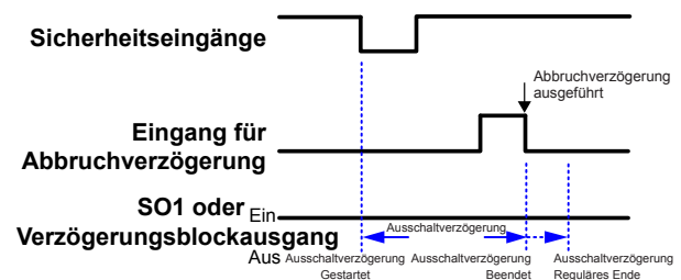
Abbildung 23. Ausgang bleibt für Sicherheitseingänge ohne Latch-Reset eingeschaltet
