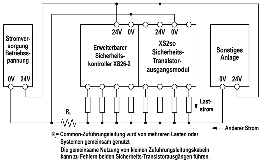
Abbildung 35. Installation des Common-Leiters
