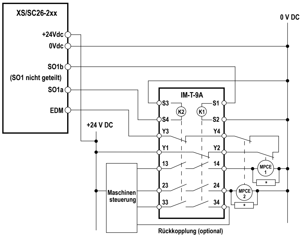
Abbildung 43. Typischer Anschluss des XS/SC26-2: Sicherheits-Relaisausgang (zweikanalig) mit EDM
