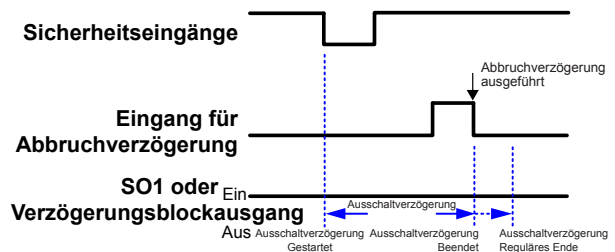
Abbildung 30. Ausgang bleibt für Sicherheitseingänge ohne Latch-Reset eingeschaltet
