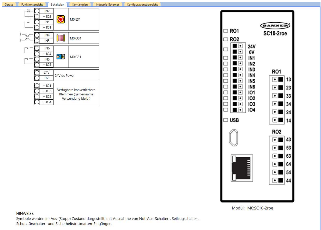
Abbildung 219. Registerkarte Schaltplan mit einem Not-Aus-Schalter, optischen Sensor und Schutztürschalter
