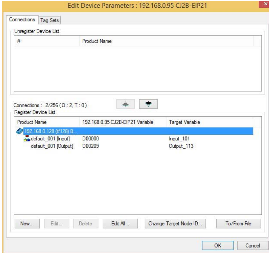
Abbildung 186. Fenster Parameter bearbeiten
