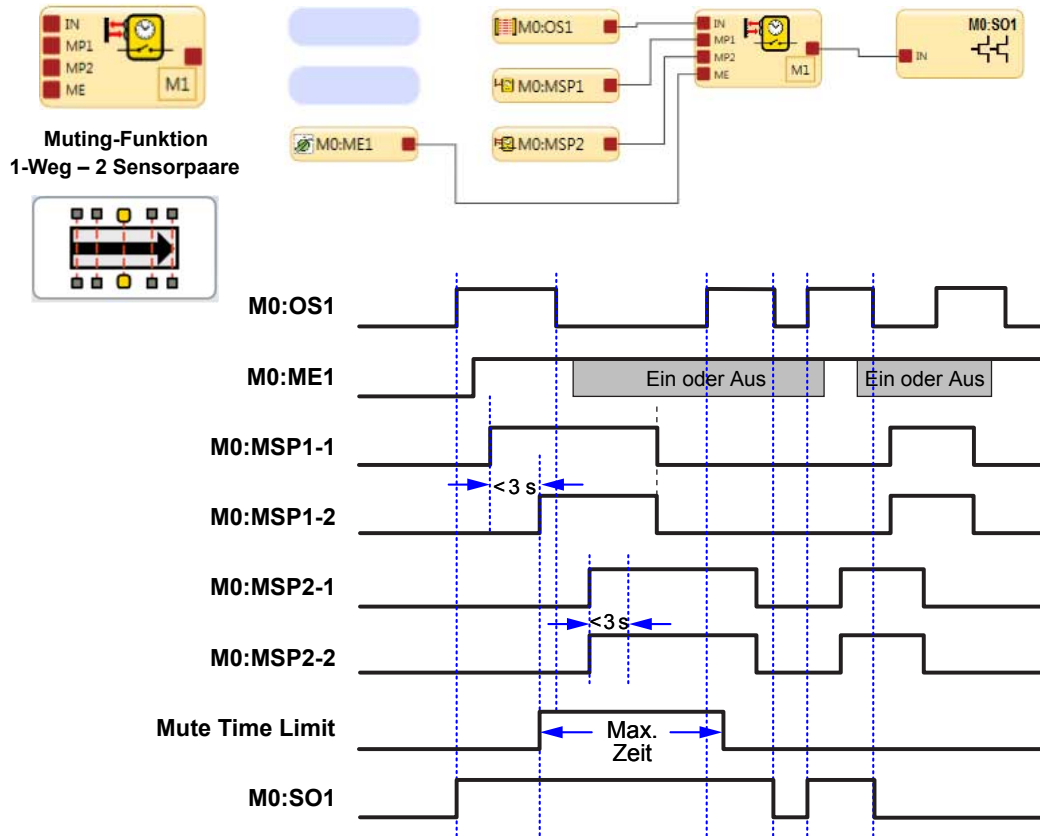
Abbildung 78. Zeitablauf-Diagramm: Unidirektionaler Muting-Block, zwei Muting-Sensorpaare
