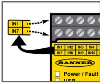
Abbildung 15. Position der Eingangs- und Ausgangsanschlüsse am XS/SC26-2
