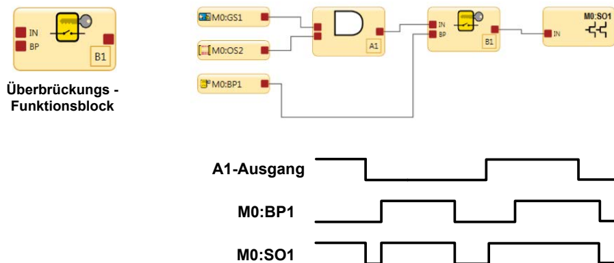
Abbildung 63. Zeitablauf-Diagramm: Überbrückungsblock
