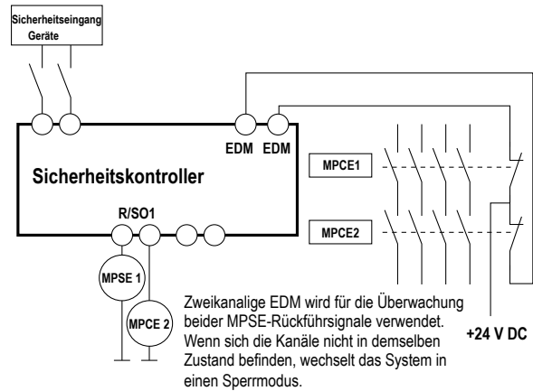
Abbildung 38. Anschluss der externen Zweikanal-Geräteüberwachung (Zweikanal-EDM)
