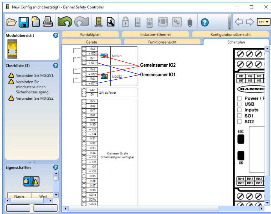
Abbildung 5. Registerkarte Schaltplan – Ansicht gemeinsam genutzter Ein-/Ausgänge
