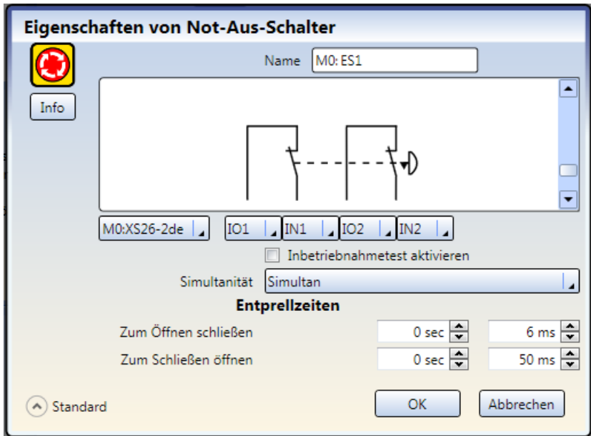
Abbildung 50. Erweiterte Einstellungen für Sicherheitseingänge
