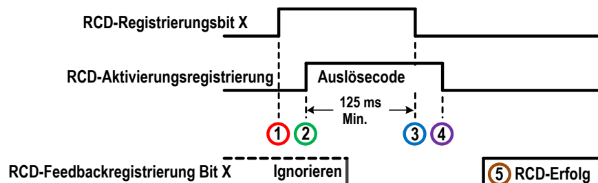
Abbildung 26. Virtuelle Reset- oder Abbruchverzögerungssequenz (RCD) - zeitgeschaltete Methode
