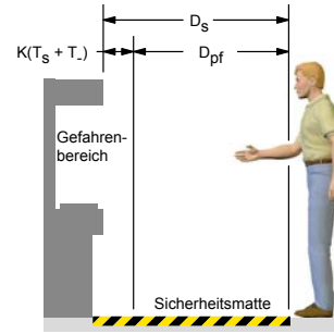
Abbildung 18. Ermittlung des Sicherheitsabstands für die Sicherheitsmatte
