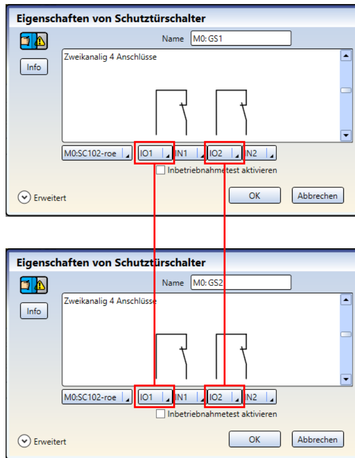
Abbildung 4. Gemeinsame Nutzung von IO1 und IO2 durch GS1 und GS2
