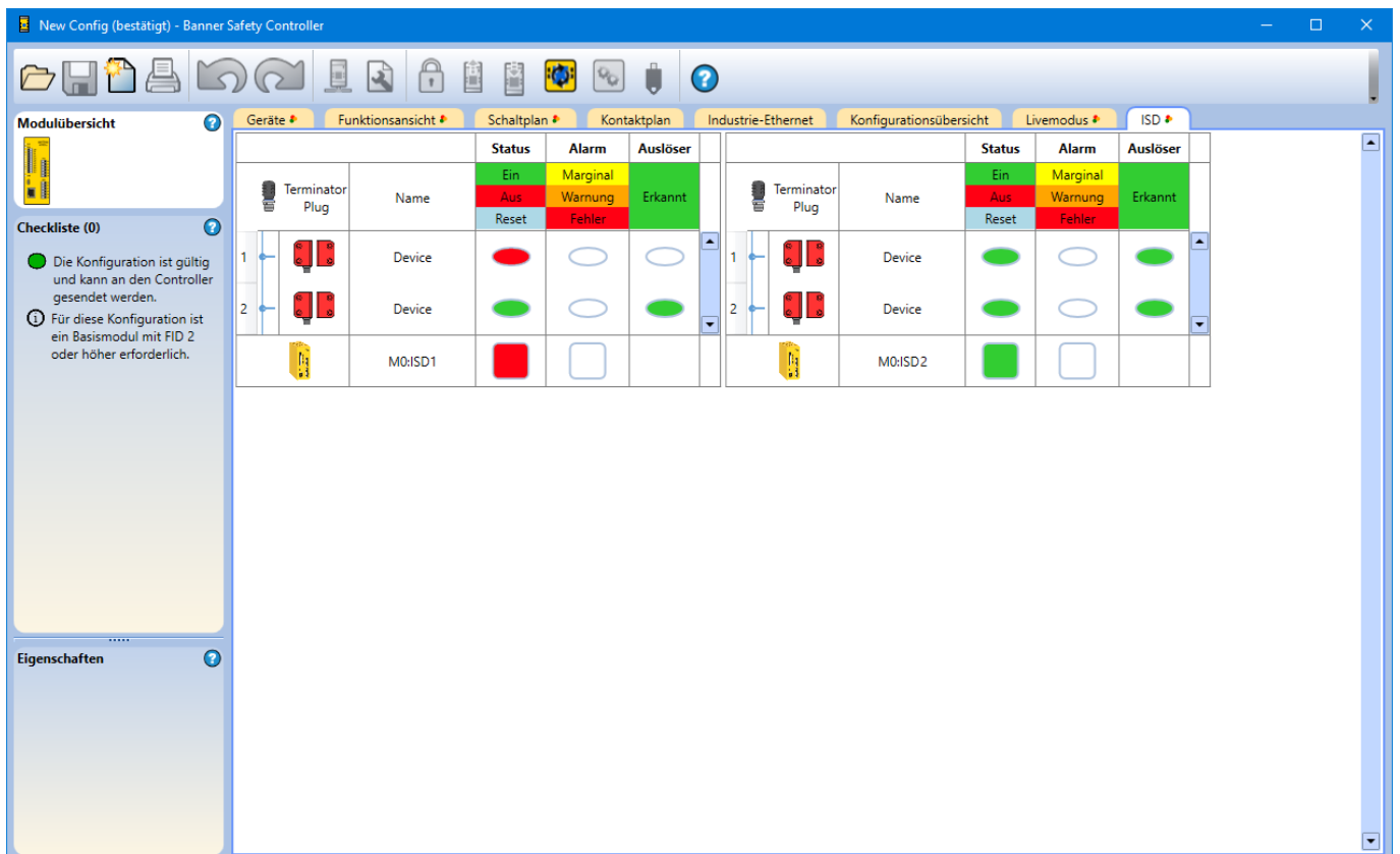
Abbildung 110. Laufzeit – SC10-2 Registerkarte ISD
