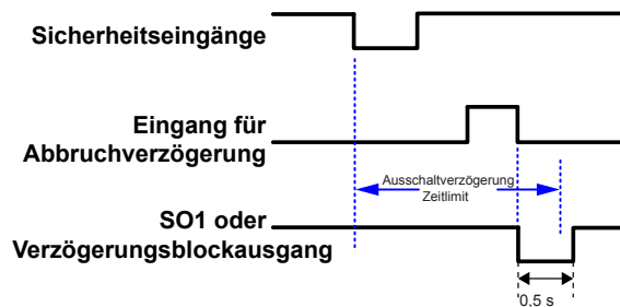
Abbildung 21. Ausgang schaltet sich aus
