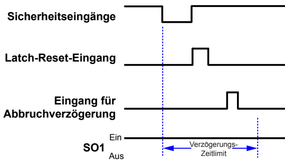
Abbildung 29. Ausgang bleibt für Sicherheitseingänge mit Latch-Reset eingeschaltet
