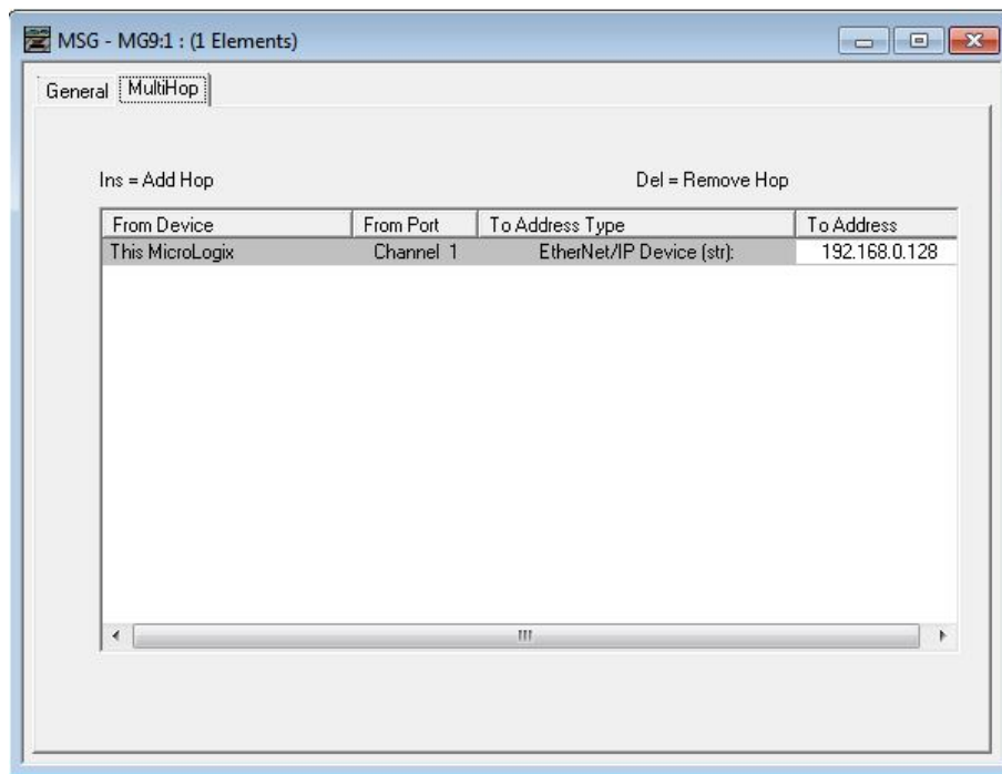
Abbildung 201. Fenster MSG - MG9:1 (1 Element) – Registerkarte MultiHop
