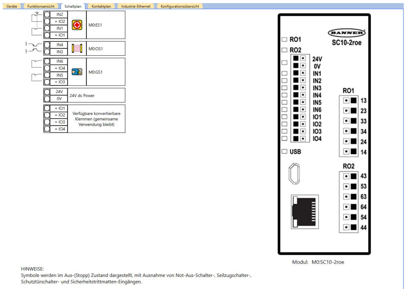
Abbildung 222. Registerkarte Schaltplan mit einem Not-Aus-Schalter, optischen Sensor und Schutztürschalter
