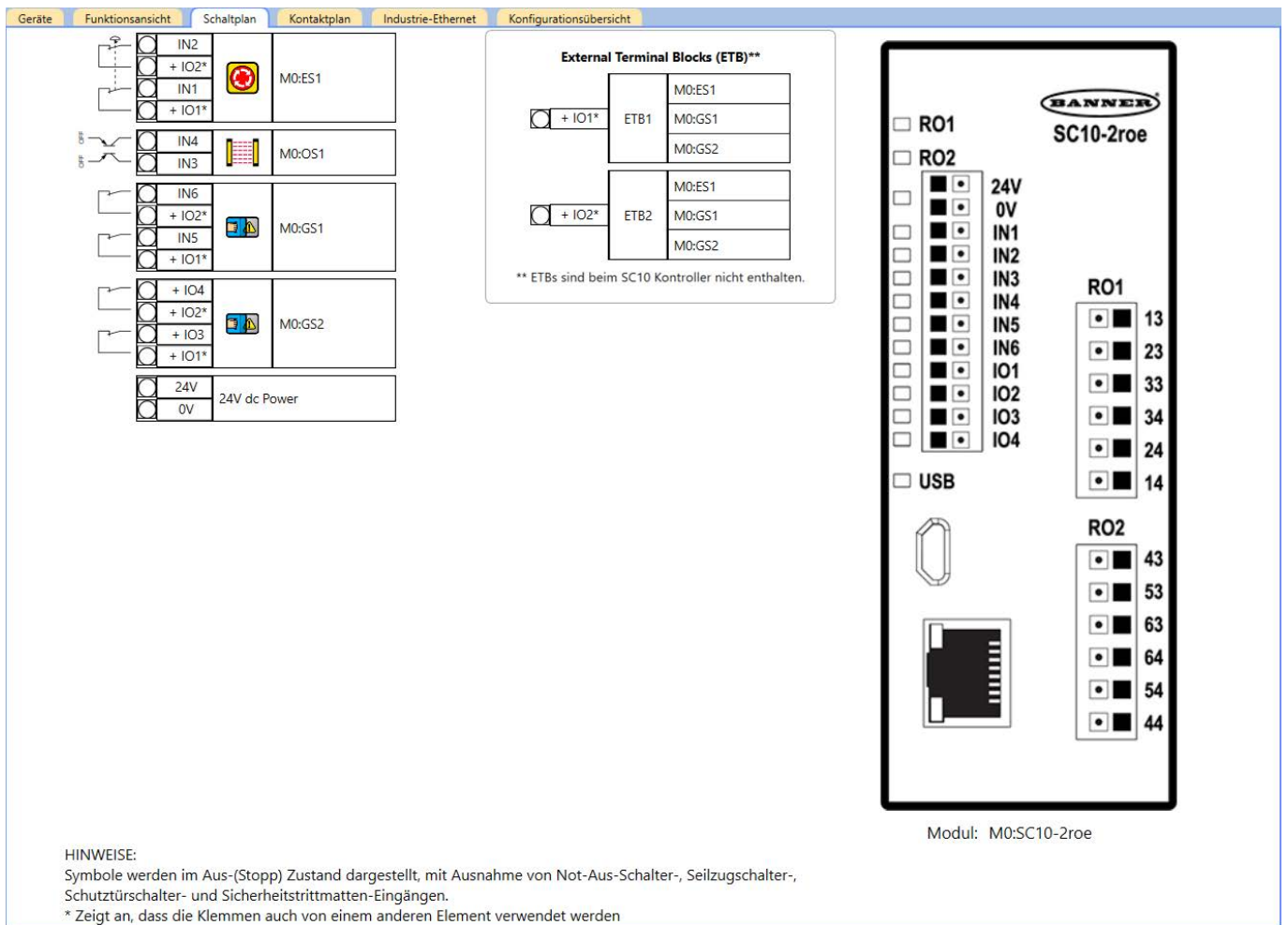
Abbildung 90. Registerkarte Schaltplan : SC10-2 mit externen Klemmenblöcken
