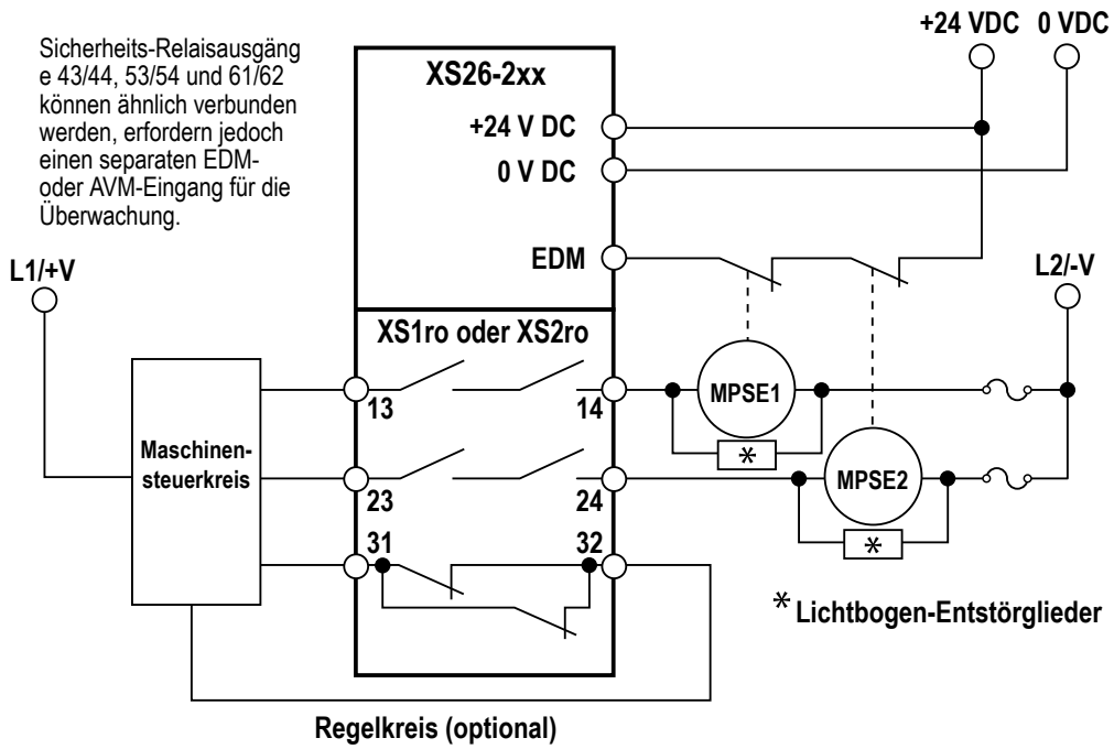
Abbildung 43. Typischer Anschluss des XS/SC26-2: Sicherheits-Relaisausgang (zweikanalig) mit EDM
