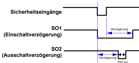
Abbildung 31. Zeitablauf-Diagramm: Ein- und Ausschaltverzögerung für Sicherheitsausgänge allgemein
