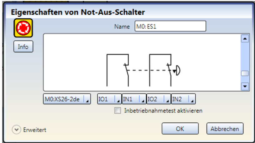
Abbildung 49. Allgemeine Einstellungen für Sicherheitseingänge
