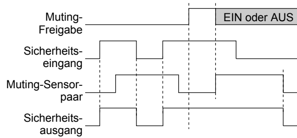
Abbildung 82. Zeitgebungslogik: ein Muting-Sensorpaar mit Muting-Freigabe
