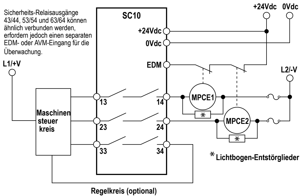
Abbildung 45. Typischer Anschluss des SC10-2: Sicherheits-Relaisausgang (zweikanalig) mit EDM
