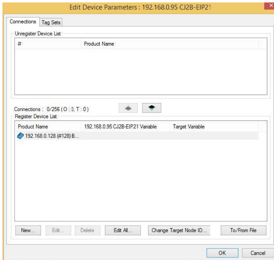
Abbildung 184. Fenster Geräteparameter bearbeiten – Registerkarte Verbindungen
