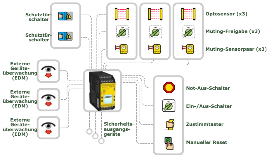
Abbildung 54. Beispielkonfiguration (schematische Darstellung)
