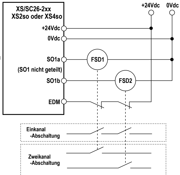
Abbildung 42. Typischer Anschluss des XS/SC26-2: Sicherheits-Transistorausgang mit EDM
