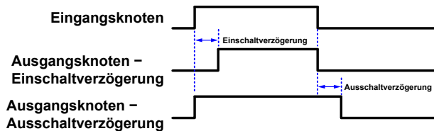
Abbildung 64. Zeitablaufdiagramm für Verzögerungsblock
