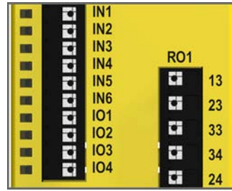
Abbildung 16. Position der Eingangs- und Ausgangsanschlüsse am SC10-2
