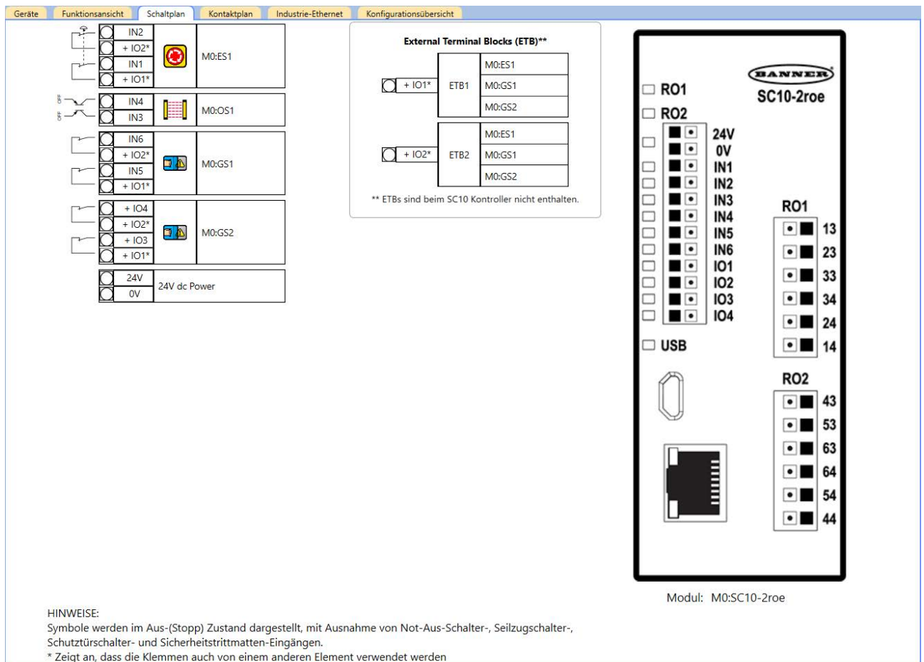
Abbildung 220. Registerkarte Schaltplan mit drei Not-Aus-Tastern und ETBs
