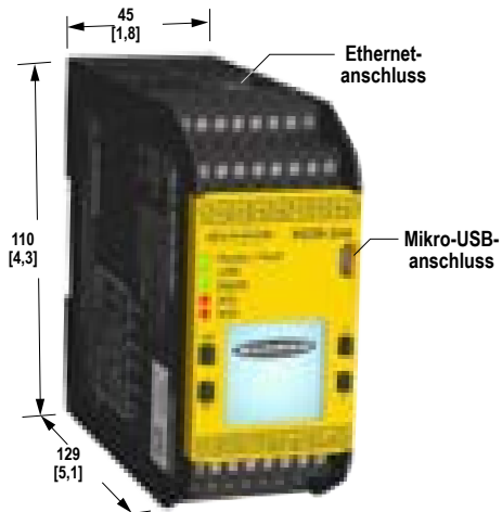
Abbildung 10. XS/SC26-2 Basismodul – Abmessungen
