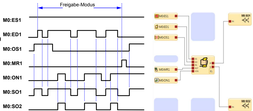
Primärer Zustimmtaster & Sekundäre Ausgangssteuerung
