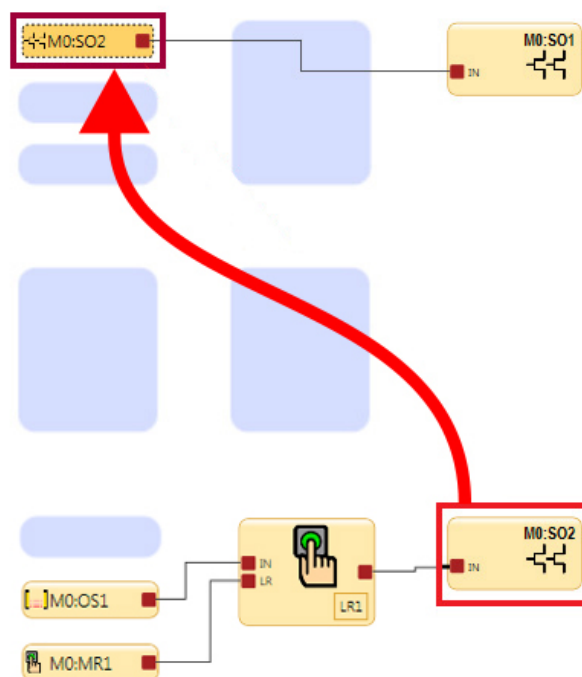
Abbildung 119. Von einem anderen Sicherheitsausgang gesteuerter Sicherheitsausgang
