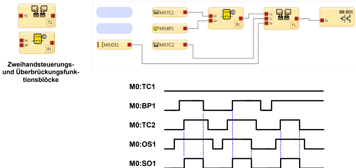
Abbildung 83. Zeitablauf-Diagramm: Zweihandsteuerungsblock
