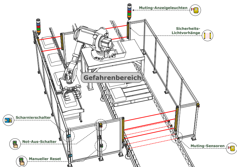
Abbildung 13. Anwendungsbeispiel: Roboterzelle
