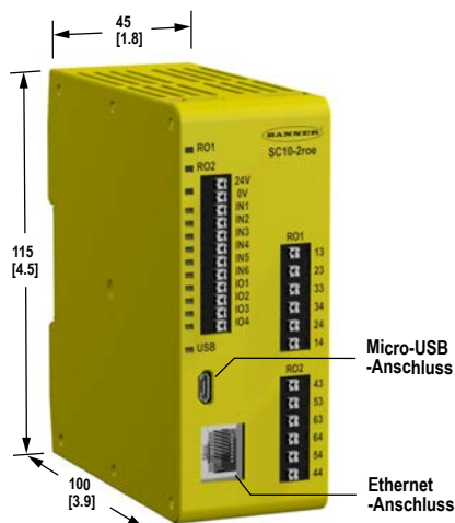
Abbildung 12. Abmessungen des SC10-2
