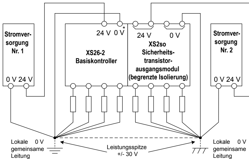
Abbildung 36. Schaltplan – Empfohlene Erdung
