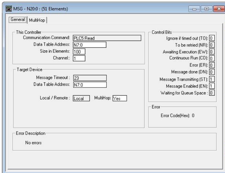
Abbildung 198. Fenster MSG - N20:0 (51 Elemente) – Registerkarte Allgemein
