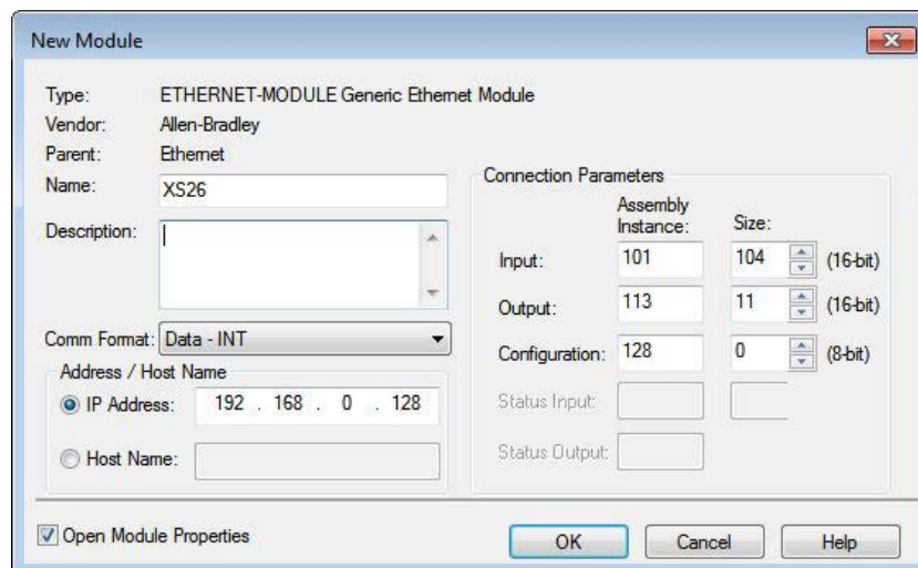
Abbildung 148. SPS-Eingang Baugruppe 101 (0x65), Größe 104 Wörter (VI-Fehlerindexwörter)
