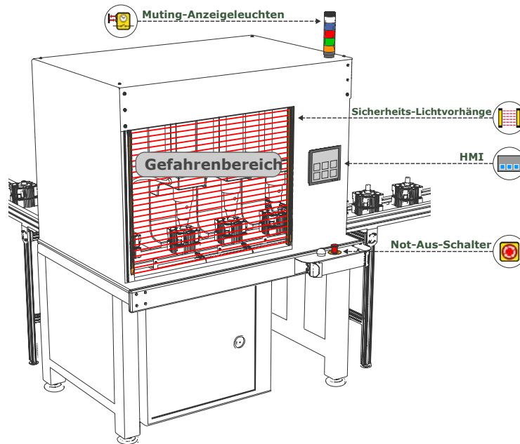
Abbildung 14. Anwendungsbeispiel für den SC10-2
