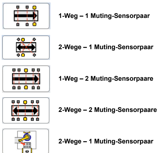
Abbildung 73. Muting-Block: Funktionsarten
