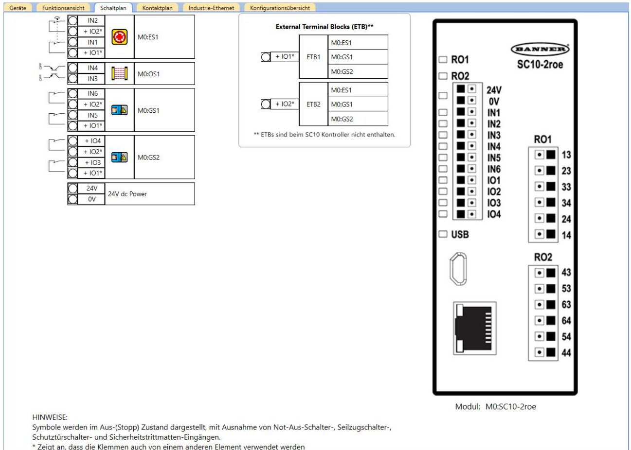
Abbildung 225. Registerkarte Schaltplan mit Not-Aus-Schalter, optischen Sensor, Schutztürschaltern und ETBs
