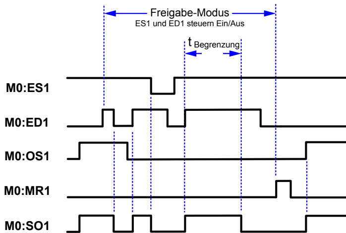
Abbildung 66. Zeitablauf-Diagramm: Zustimmtaster, einfache Konfiguration
