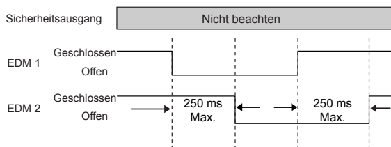
Abbildung 40. Zeitgebungslogik: Zweikanalige EDM, zeitliche Abstimmung zwischen Kanälen
