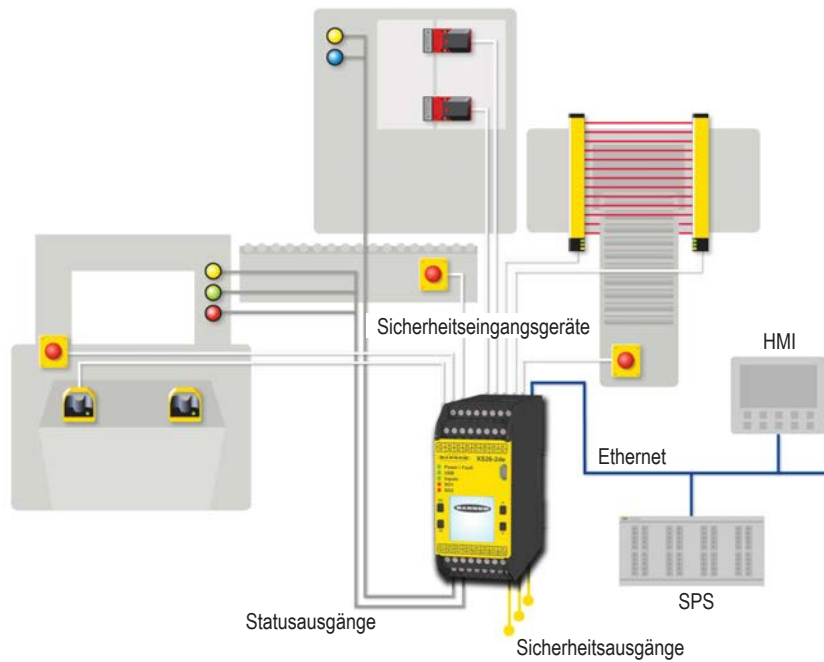
Abbildung 3. Sicherheitsausgänge (Beispielanwendung)
