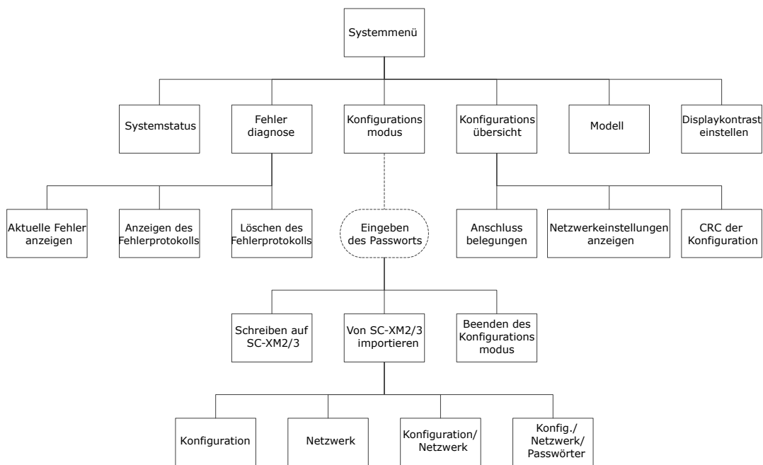
Abbildung 120. Bedienfeld am Controller: Zuordnung
