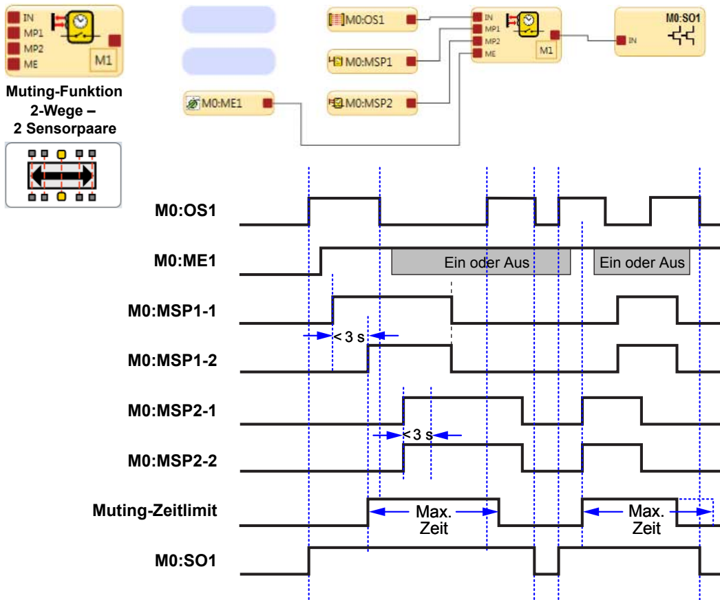
Abbildung 80. Zeitablauf-Diagramm: Bidirektionaler Muting-Block, zwei Muting-Sensorpaare
